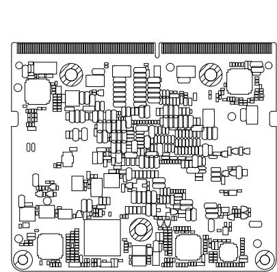
BOTTOM PCBA
