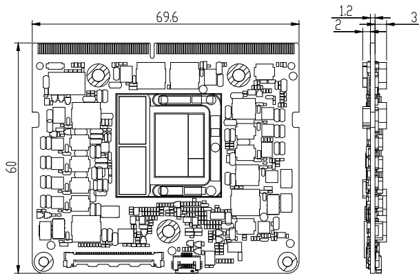
TOP PCBA View Scale: 1:1
